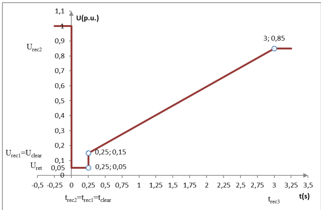
4.att. B tipa parka moduļa bojājumnoturības profils
