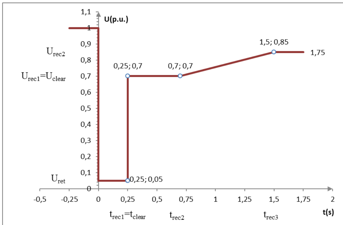
3.att. B tipa sinhrona moduļa bojājumnoturības profils,
